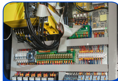
QUADRO ELÉTRICO
